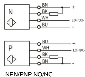
NPN/PNP NO/NC
