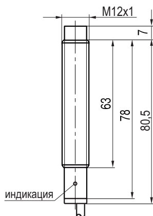
Габаритный чертеж
