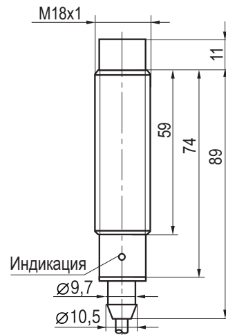
Габаритный чертеж
