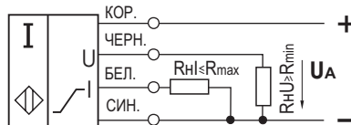
Схема подключения с пропорциональным выходным напряжением
