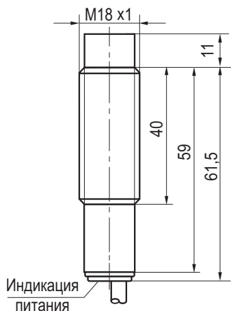
Габаритный чертеж
