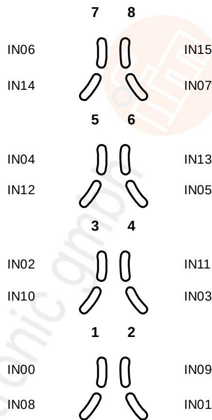
Grafik: LEDs für Status der Eingänge
