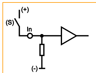
Prinzipialschaltung Binäreingang plus-schaltend (BL) für positives Sensorsignal: Eingang = offen \Rightarrow Signal = Low (GND)
