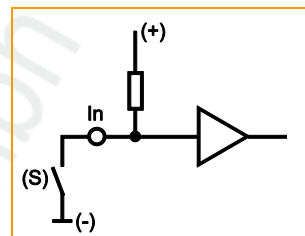
Prinzipialschaltung Binäreingang minus-schaltend (BH) für negatives Sensorsignal: Eingang = offen \Rightarrow Signal = High (Supply)
