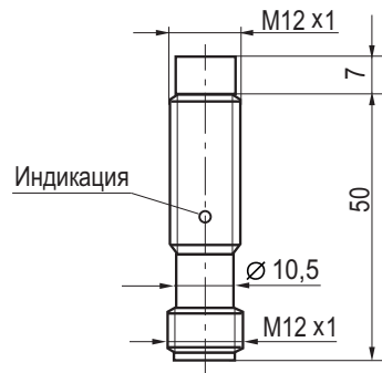
Габаритный чертеж
