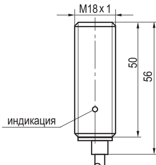
Габаритный чертеж.
