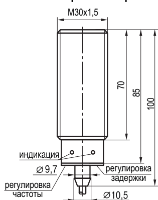
Габаритный чертеж
