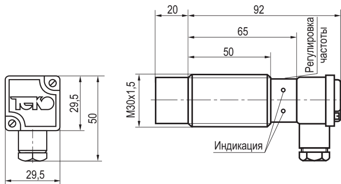
Габаритный чертеж
