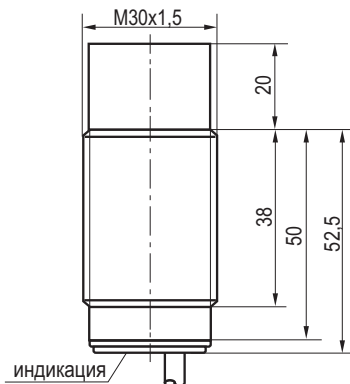
Габаритный чертеж
