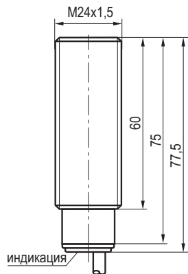
Габаритный чертеж
