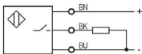
PNP NO
