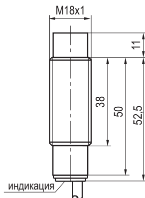
Габаритный чертеж
