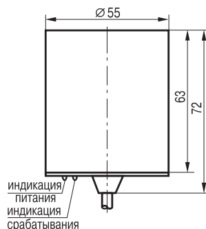
Габаритный чертёж
