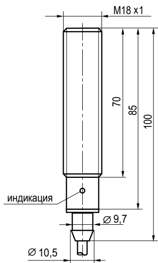
Габаритный чертеж.
