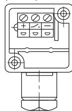
Маркировка клемм
