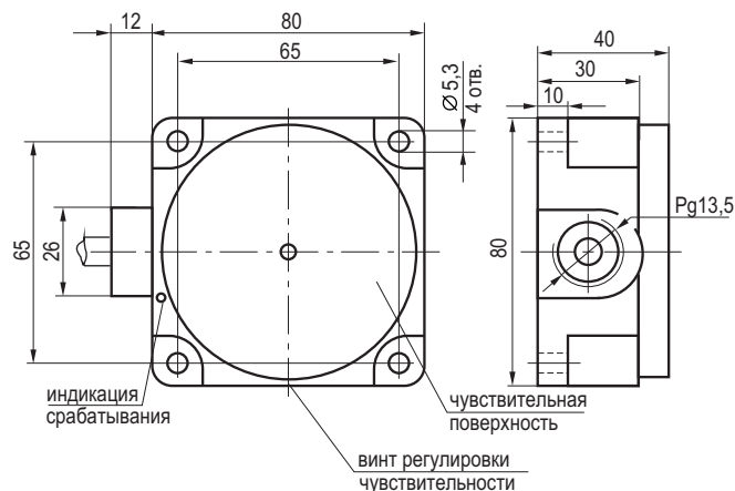
Габаритный чертеж
