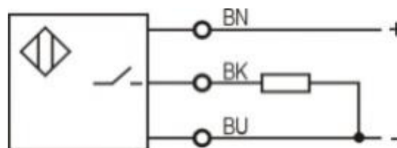
PNP NO
