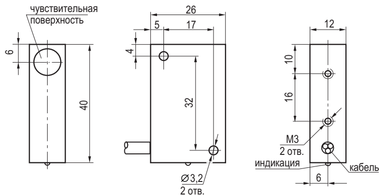
Габаритный чертеж
