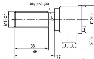
Габаритный чертеж
