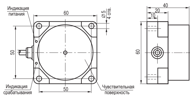
Габаритный чертеж
