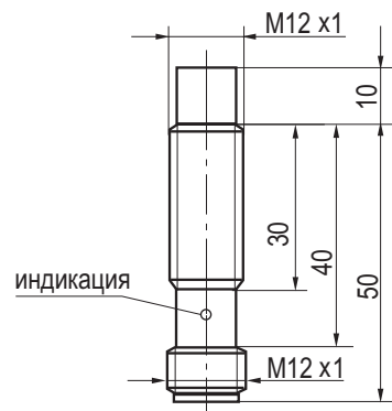
Габаритный чертеж
