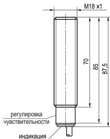
Габаритный чертеж
