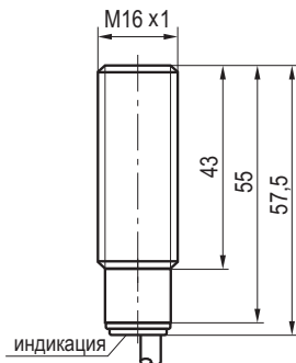
Габаритный чертеж
