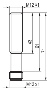
Габаритный чертеж
