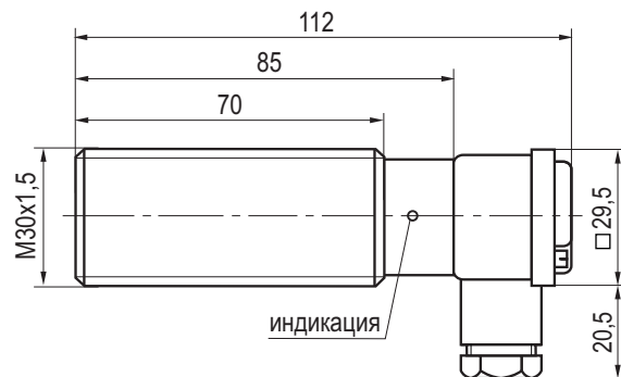
Габаритный чертеж
