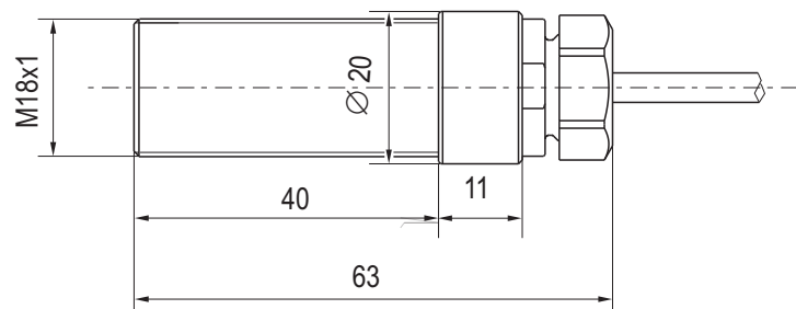
Габаритный чертеж
