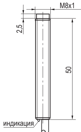
Габаритный чертеж
