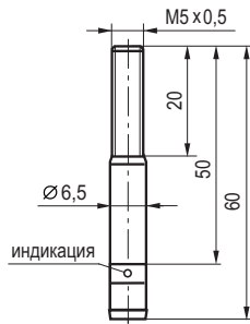
Габаритный чертеж
