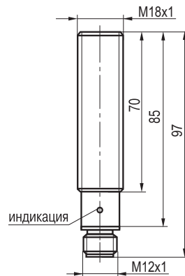
Габаритный чертеж
