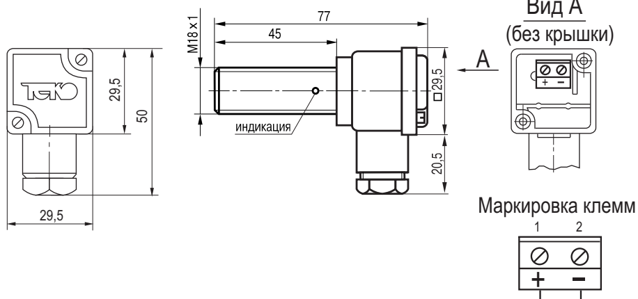
Габаритный чертеж
