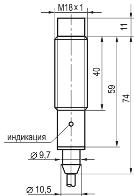
Габаритный чертеж
