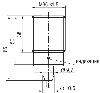
Габаритный чертеж
