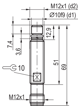
Габаритный чертеж
