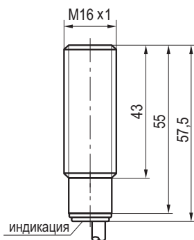
Габаритный чертеж
