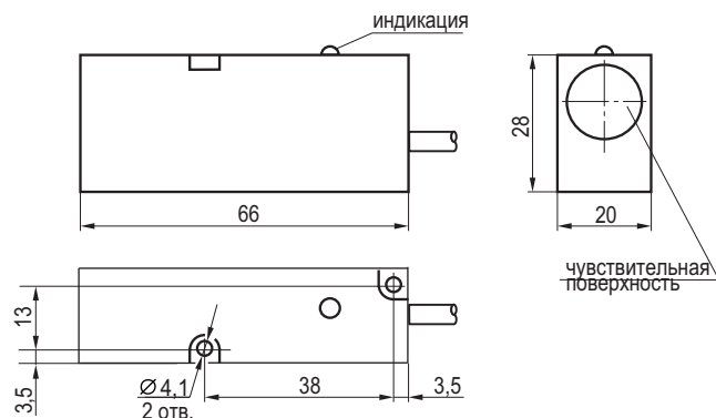
Габаритный чертеж
