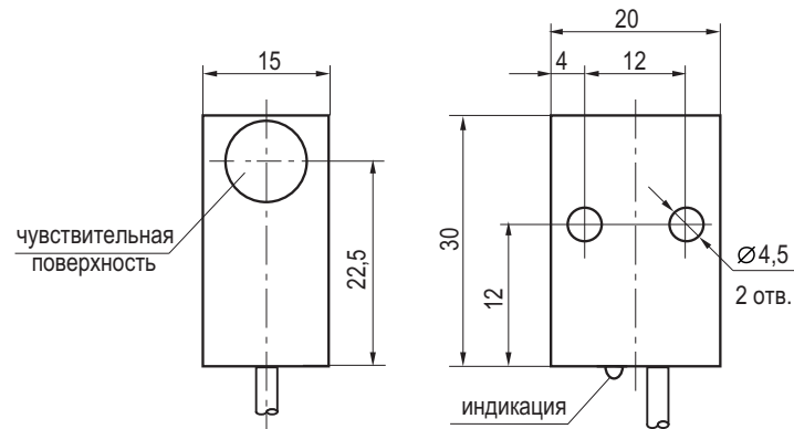
Габаритный чертеж
