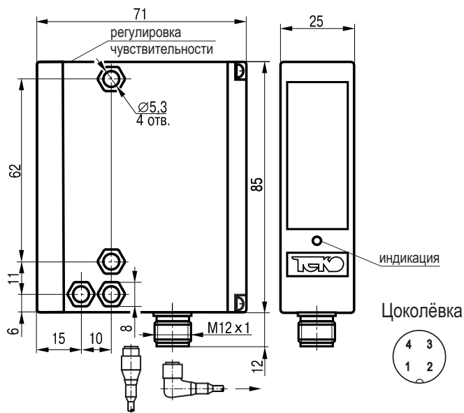
Габаритный чертеж.
