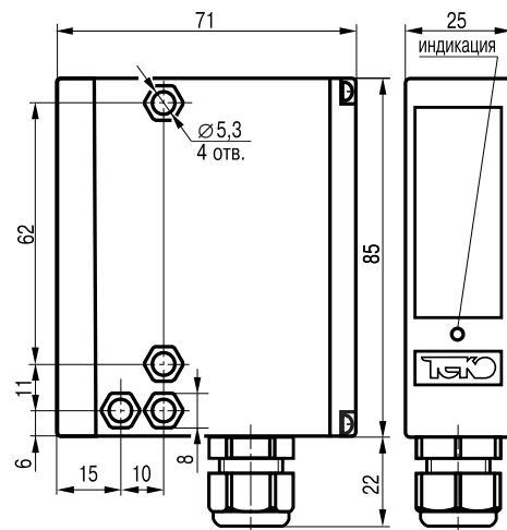
Габаритный чертеж
