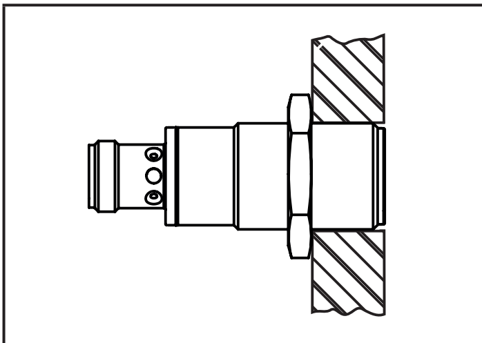
flush (DTI420)
