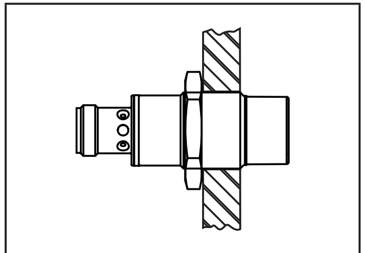
non-flush (DTI421)
