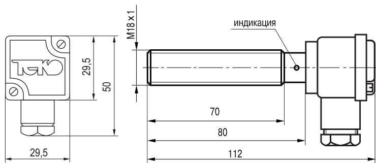
Габаритный чертеж
