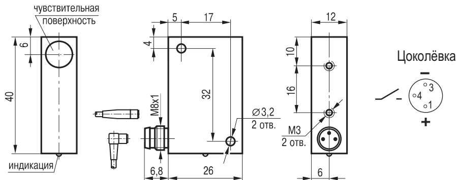
Габаритный чертеж
