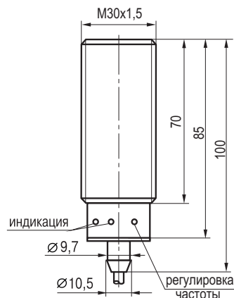
Габаритный чертеж
