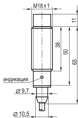
Габаритный чертеж
