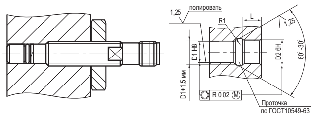
Схема монтажа
