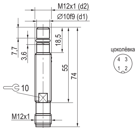
Схема монтажа
