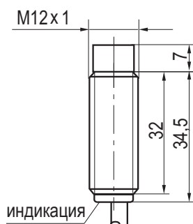
Габаритный чертеж
