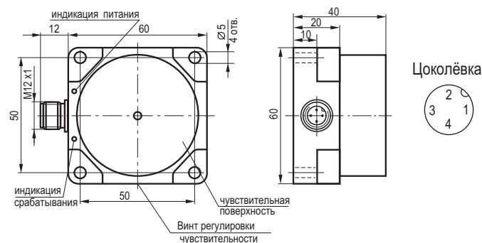
Габаритный чертеж
