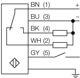
Схема подключения
