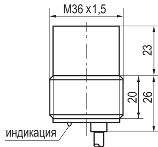
Габаритный чертеж
