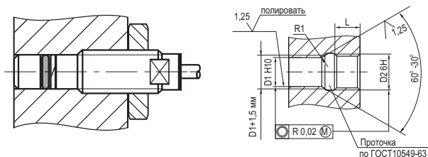
Схема монтажа
