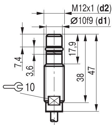
Габаритный чертеж
